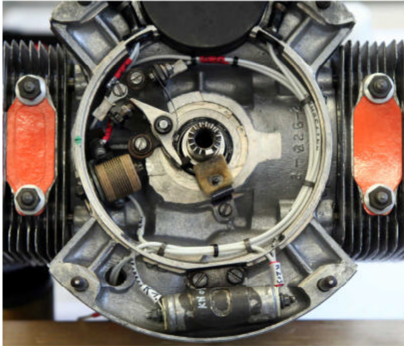
PTFE Kabel ohne Schutzschlauch ausgeführt.
